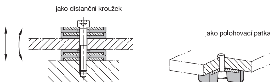
Příklad montáže
